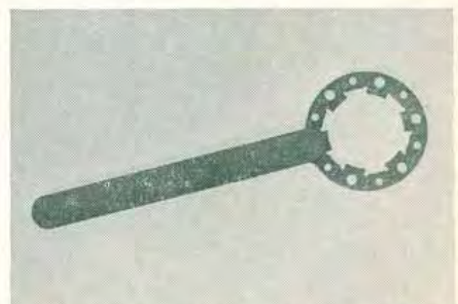
Blokkeerhaak voor koppeling Afb. 40 Onderdeelnr. 09.30.31
