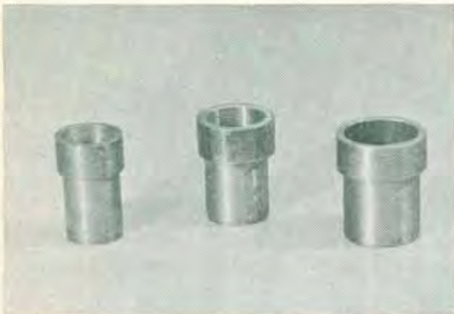
Monteerhuls voor simmeringen Afb. 35 Onderdeelnr. 15 Ø = 09.30.34 17 Ø = 09.30.11 20 Ø = 09.30.35
