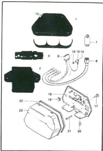
afb. 43b - overige onderdelen clignoteursset
