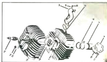
afb. 14 - cilinder, kop + zuiger
