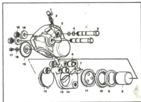
afb. 60 - schijfremklauw
