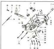
afb. 25a - carterhelpt links (indirecte schakeling)
