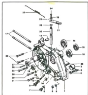
afb. 25b - carterhelft links (directe of hevelschakeling)
