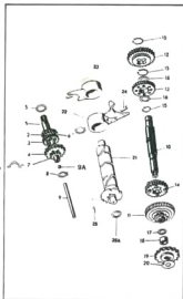
afb. 28 - 4-versnellingsbak (directe of hevelschakeling)
