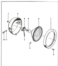
afb. 45 - koplamp
