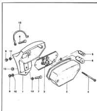
afb. 46 - achterlicht
