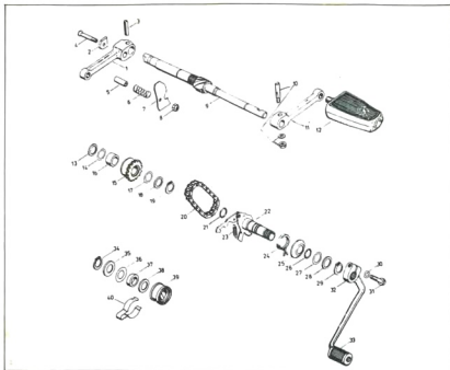
afb. 30 - trapmechanisme (4-versn., directe schakeling)
