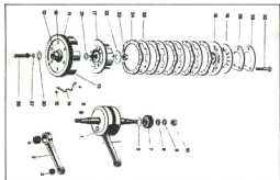
afb. 17 - krukas + koppeling
