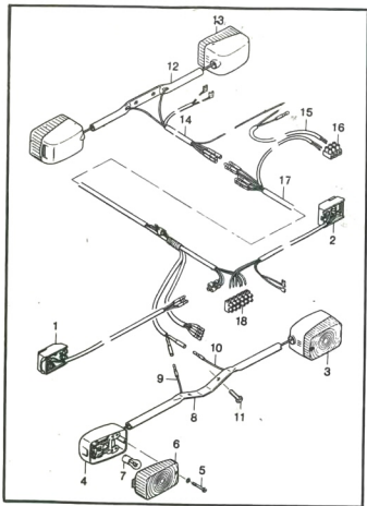
afb. 43a - clignoteurs en schakelaar
