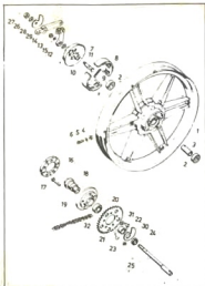
afb. 58 - achtersterwiël
