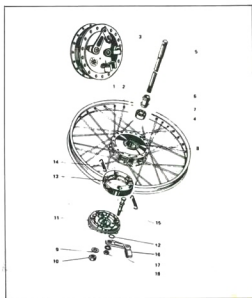
afb. 57 - voorspaakwiel
