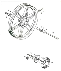
afb. 56 - voorsterwiel
