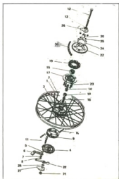
afb. 59 - achterspaakwiel
