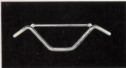
Western-Lenker , verchromt mit eingeschraubter Strebe, universal verwendbares Modell. Gesamtbreite: ca. 750 mm Best.-Nr. 907.41 DM 22,20
