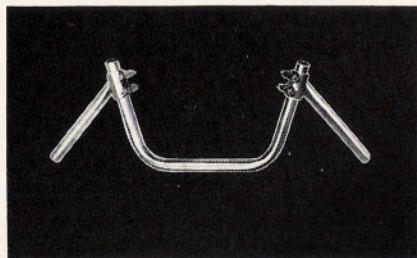
Sportlenker , 3-teilig verchromt, vielfach verstellbar und universell verwendbar. Gesamtbreite: ca. 750 mm Best.-Nr. 907.69 DM 29,80
