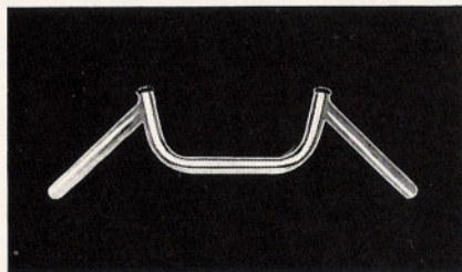
Sportlenker , Modell John Tickle verchromt, Lenkerenden herabgezogen, universell verwendbar. Gesamtbreite: ca. 540 mm Best.-Nr. 907.66 DM 18,50 mit 2 Bohrungen, passend für Zündapp-Modelle ab 1967 (Ges.-Breite 600 mm) Best.-Nr. 907.68 DM 19,80
