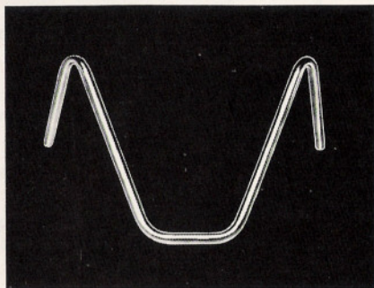
Western-Lenker extra hoch , verchromt universell verwendbar für Motorräder bis 250 ccm. Gesamtbreite ca. 780 mm Best.-Nr. 907.43 DM 18,50 mit 2 Bohrungen, passend für Zündapp-Modelle ab 1967 Best.-Nr. 907.47 DM 19,50
