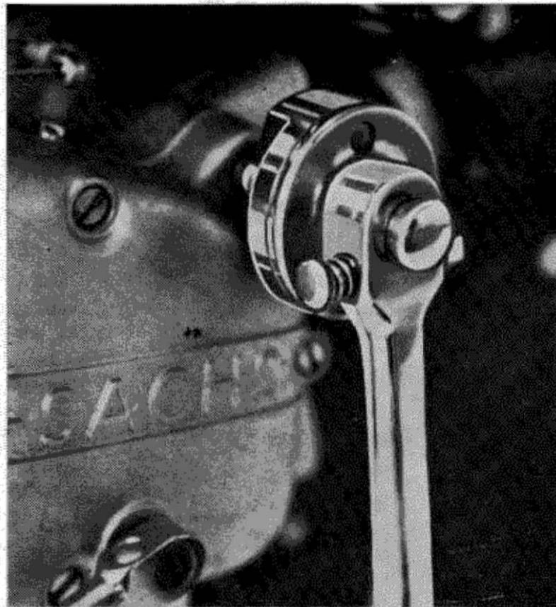
Afb. 8. Verstelbare crank
