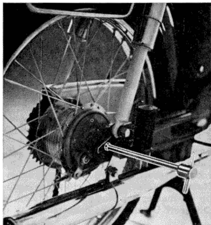
Afb. 20. Het uitnemen van het achterwiel
