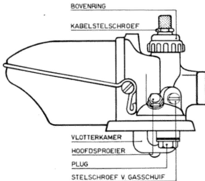
Afb. 27. De carburateur 2 versn.
