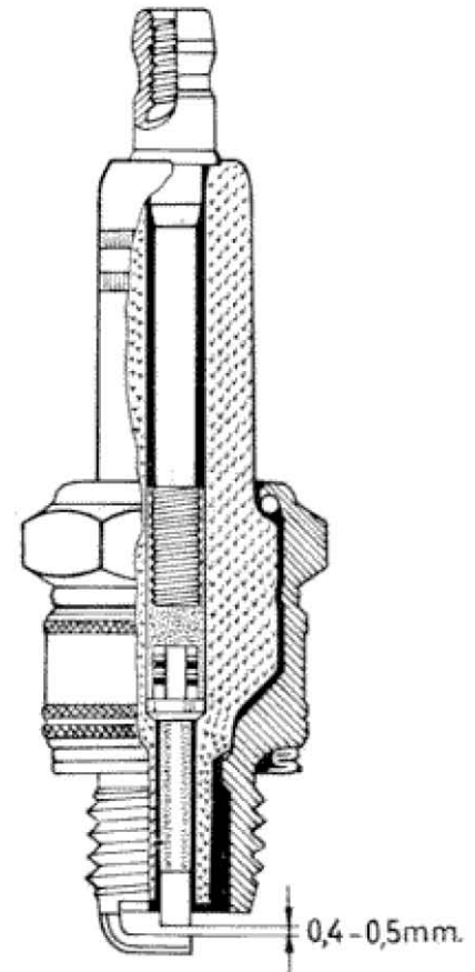
Afb. 22. De bougie
