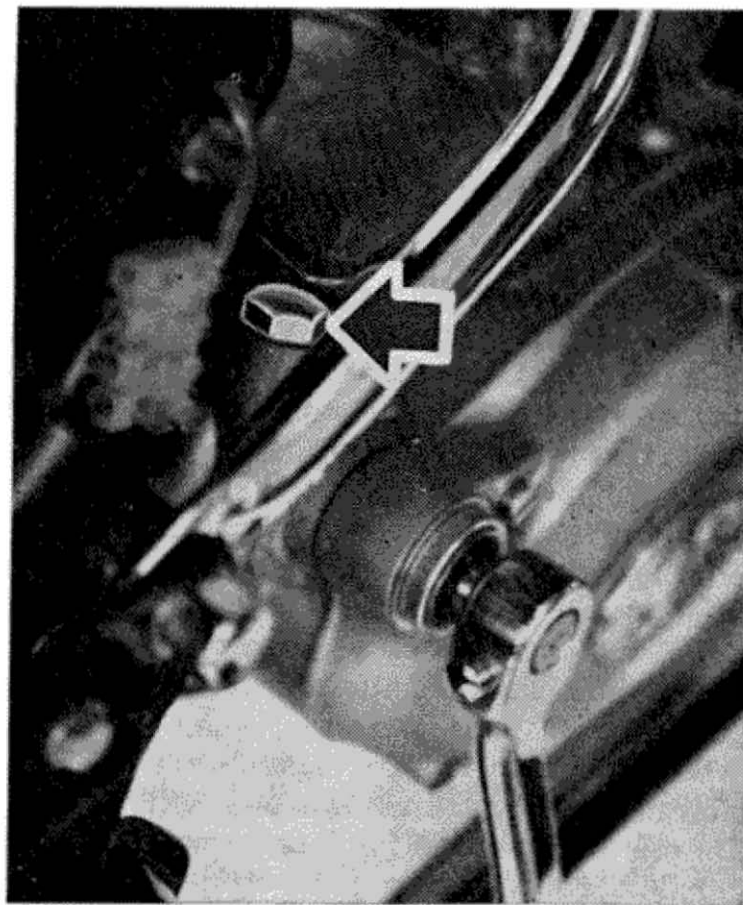
Afb. 14. Olievulschroef
