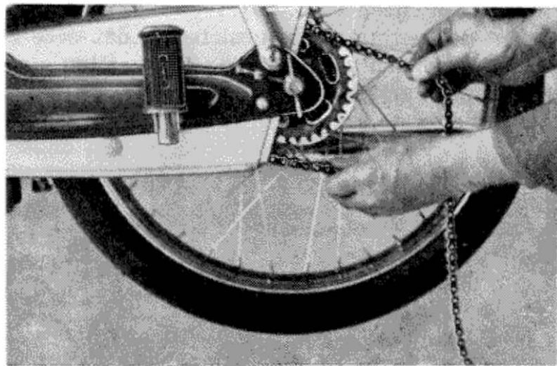
Afb. 18. Het verwisselen van de ketting
