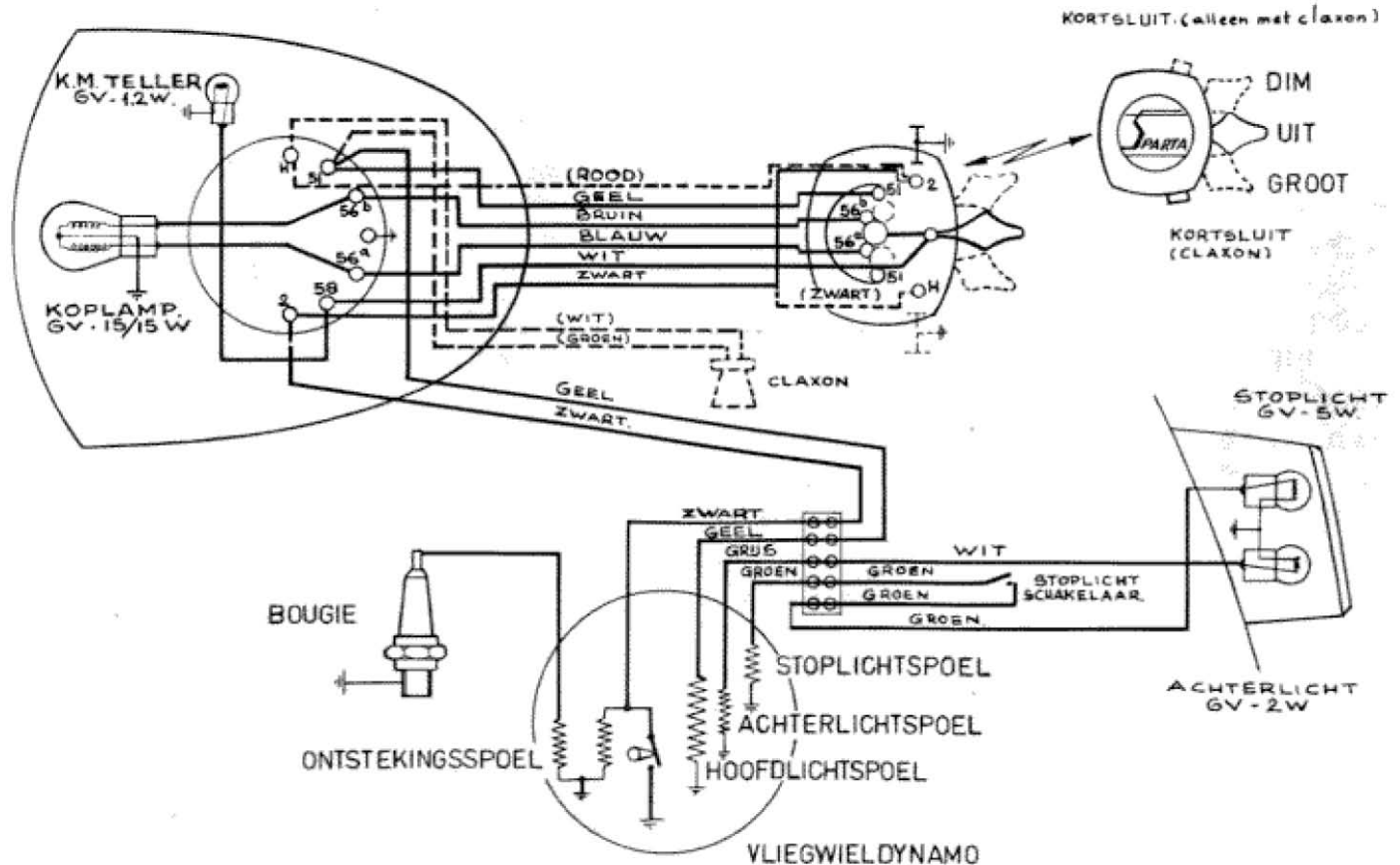
Afb. 24. Schema verlichtingsinstallatie 3 en 4 versn.
