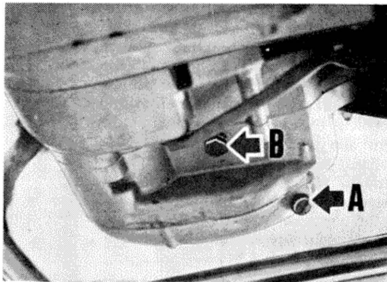
Afb. 13. A = oliecontroleschroef B = olieaftapschroef
