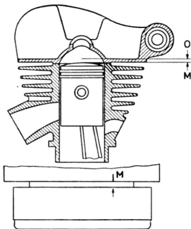
Afb. 25. O = bovenste dode punt M = moment van ontsteking
