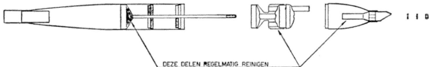
Afb. 21. De doorvoergaten, alsmede het uitneembare achterstuk behoren van tijd tot tijd gereinigd te worden
