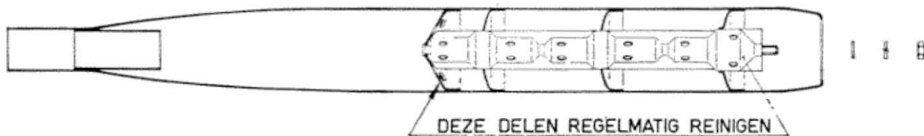
Afb. 21a. De demontabele binnenpijp en het vaste schotje in de demper behoren van tijd tot tijd gereinigd te worden
