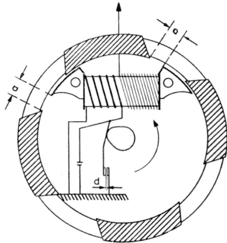
Afb. 26. Poolschoenafstand
