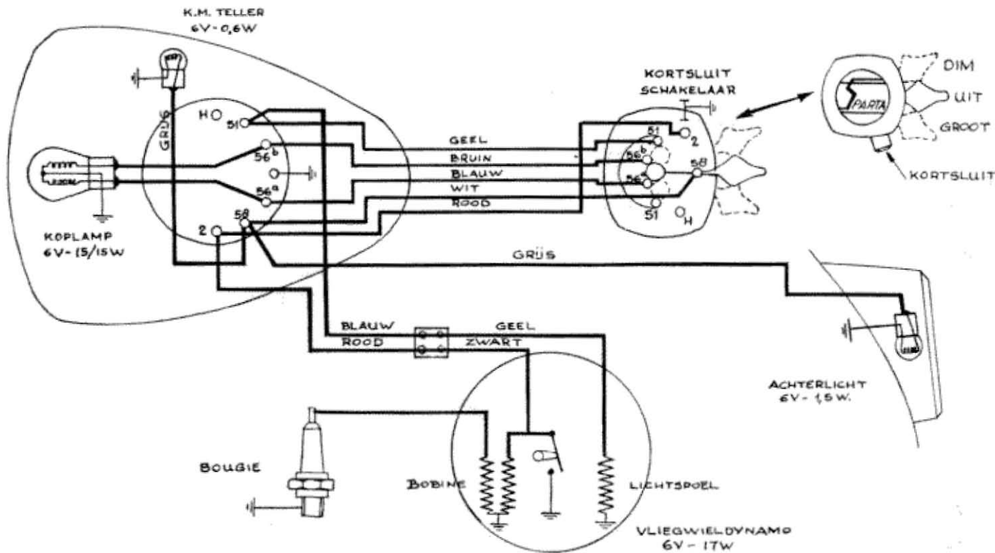
Schema verlichtingsinstallatie 2 versn. Afb. 23
