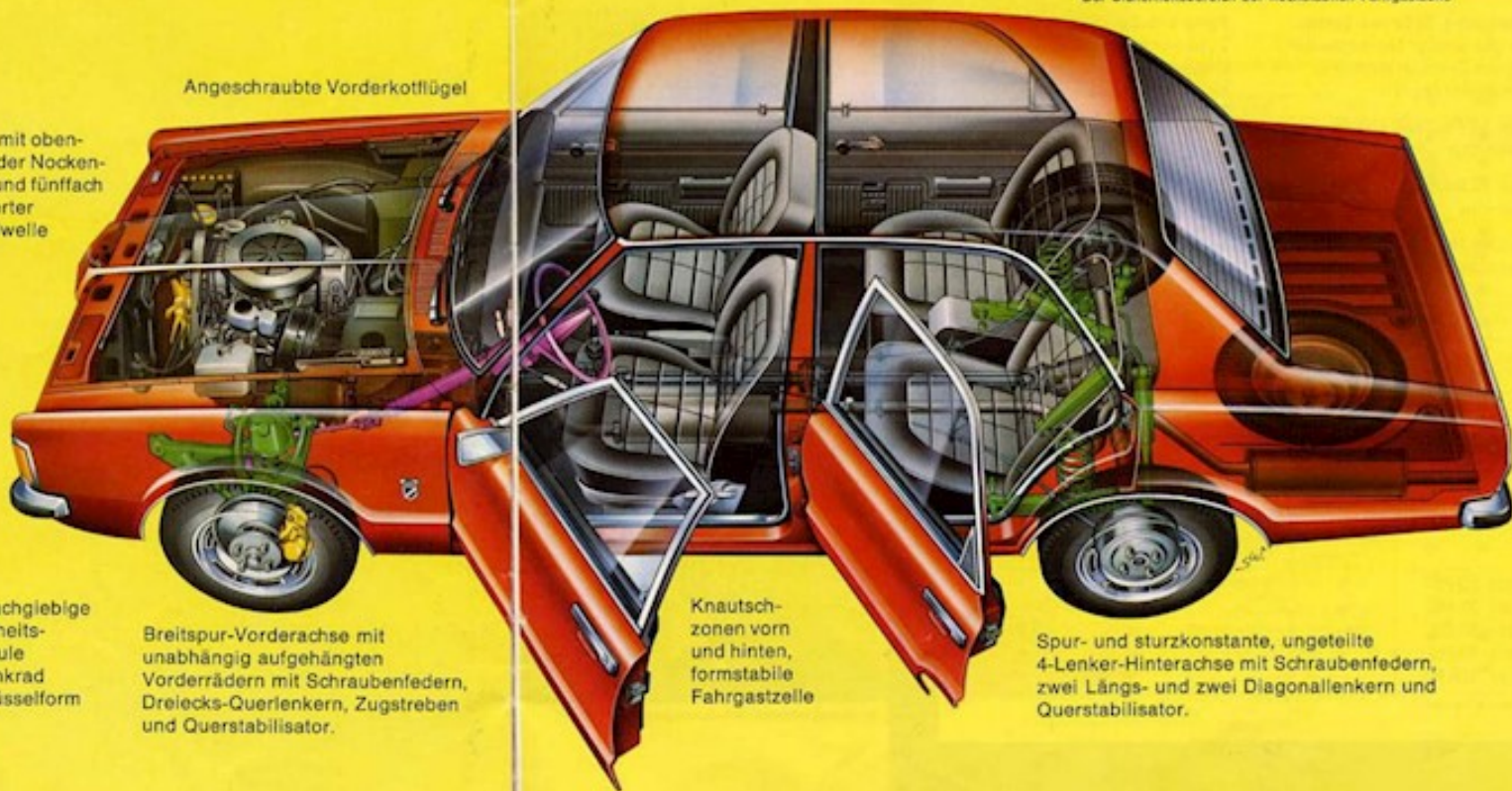
Der Sicherheitsbereich der hochstabilen Fahrgastzelle
